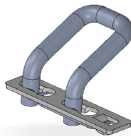
Entwurf für Zurrring, belastbar bis 2,5 t
